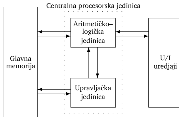
Slika 1: Struktura IAS računara
