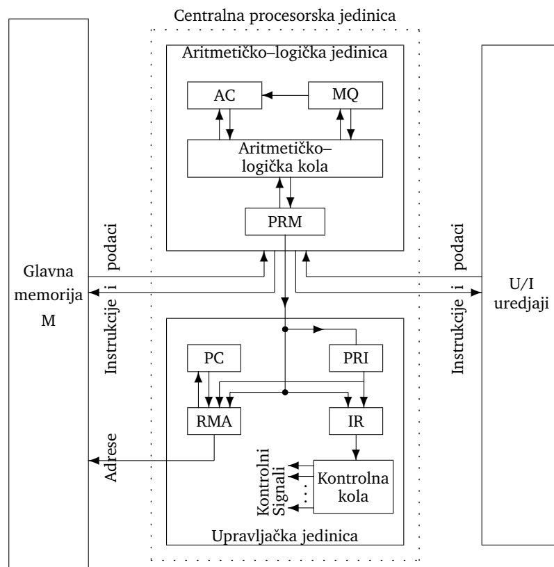
Slika 2: Detaljnija struktura IAS računara
